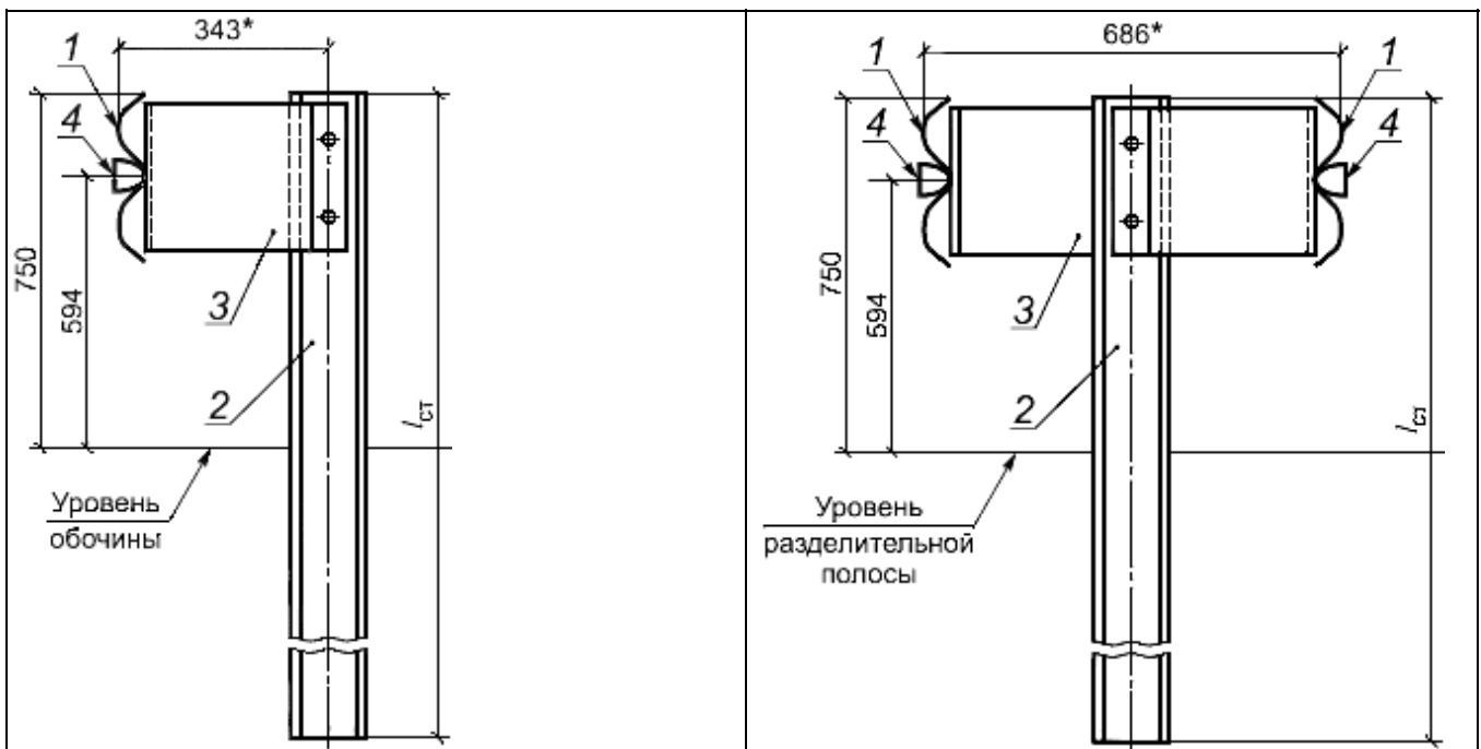
а) Одностороннее одноярусное ограждение б) Двухстороннее одноярусное ограждение
