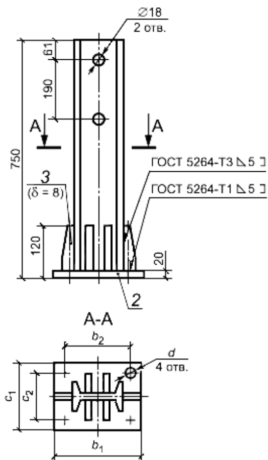
Рисунок 9 - Консоль-распорка КР
