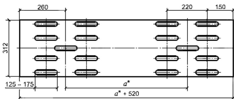
Рисунок 5 - Секция балки угловой СБУ
