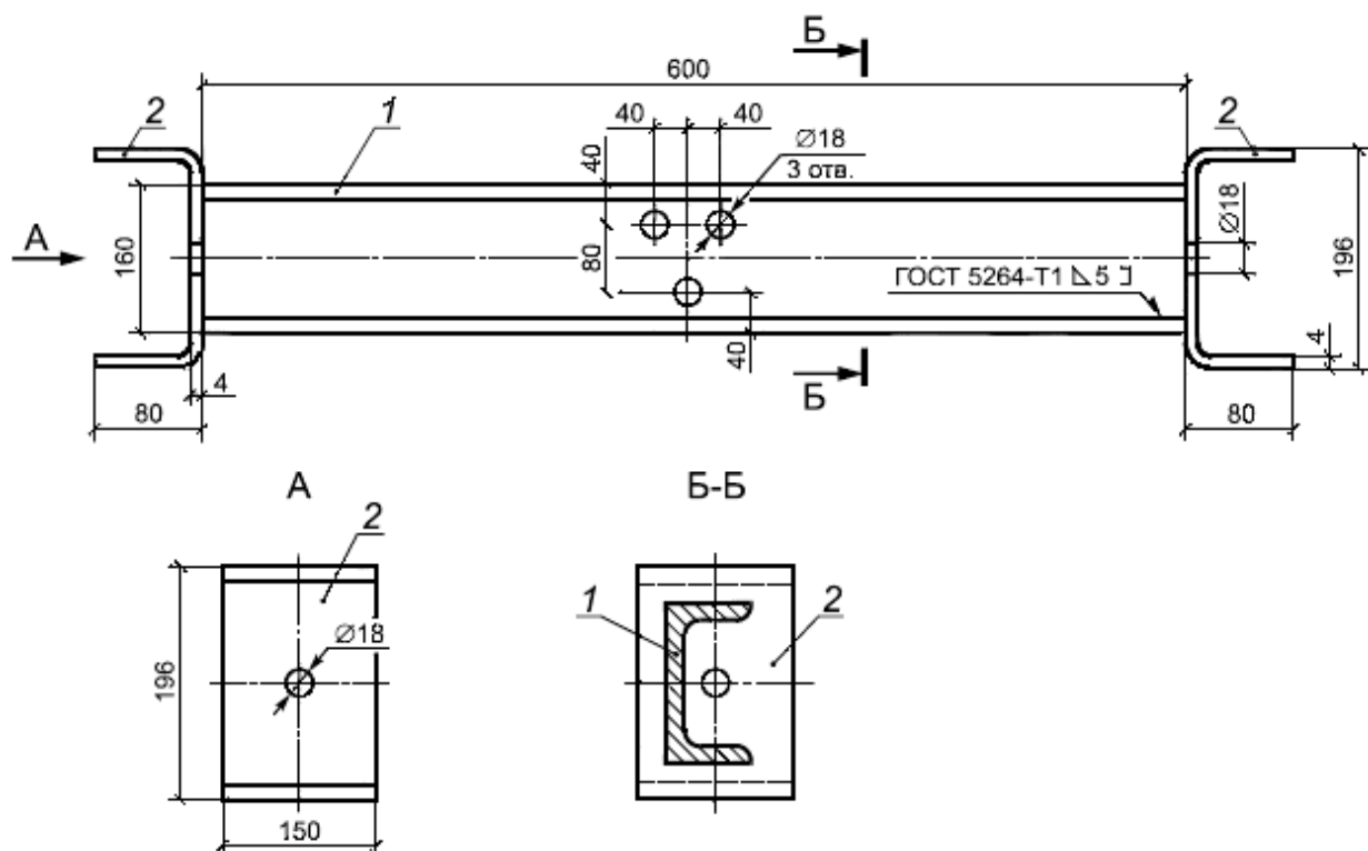
Рисунок 8 - Консоль жесткая КЖ
