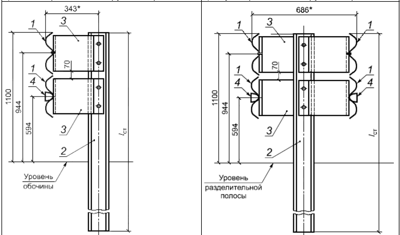
в) Одностороннее двухъярусное ограждение г) Двухстороннее двухъярусное ограждение
